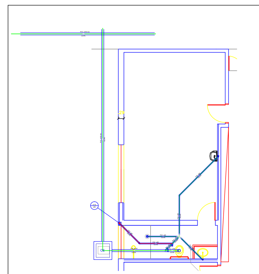
Detalhe S8 Escala 1:50
